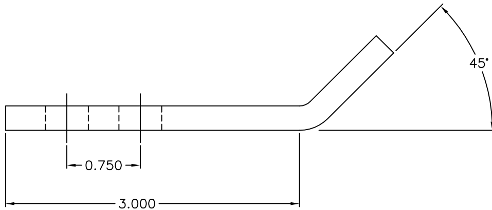
TINNED WELD LUG
